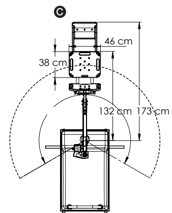
C TOP VIEW VISTA SUPERIOR VUE DE DESSUS DRAUFSICHT VISTA DALL'ALTO
