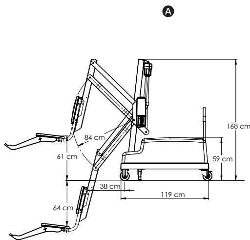
A SIDE VIEW VISTA LATERAL VUE DE CÔTÉ SEITENANSICHT VISTA LATERALE
